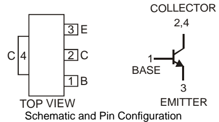
SOT89-3L
